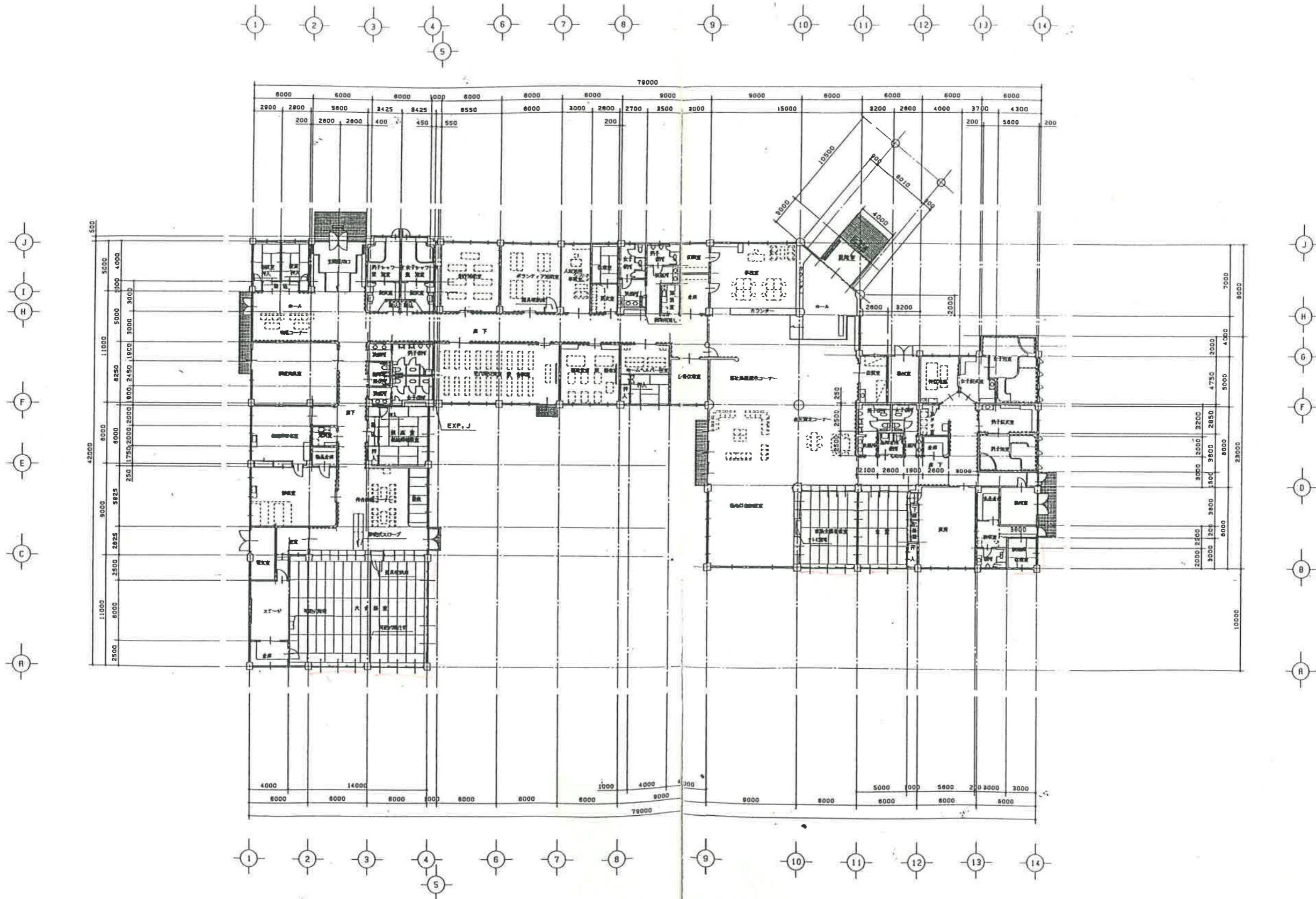
本館 平面図 1/200
