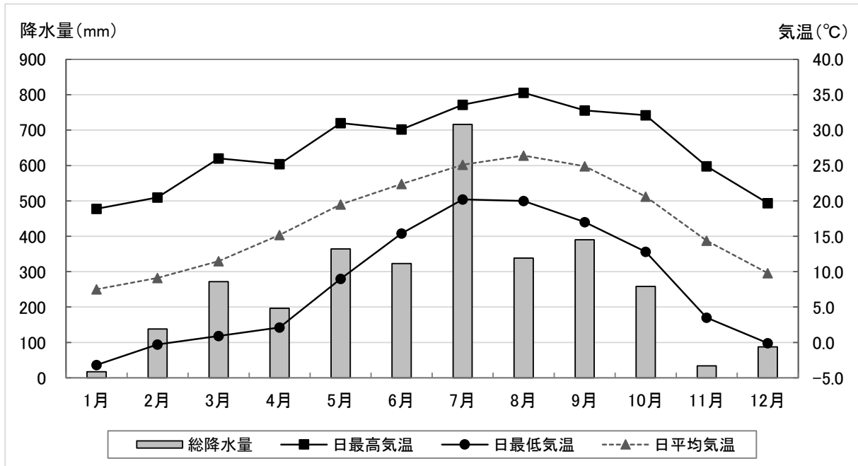
図2-1-2 気象概況（2019年）
