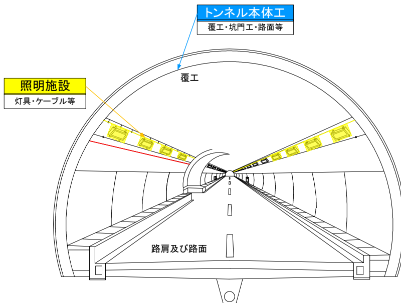
図 2.2 トンネル各施設の名称
