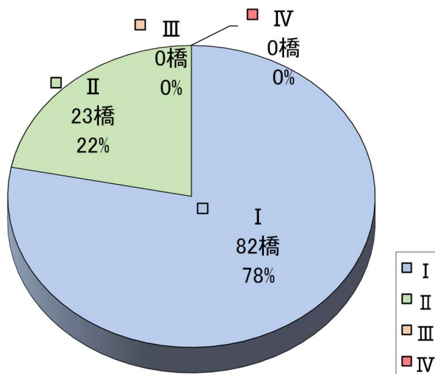
図 4 健全性の診断状況
