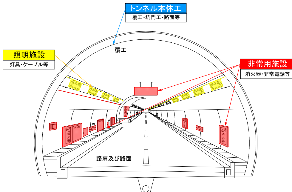
図 2.1 トンネル各施設の名称
