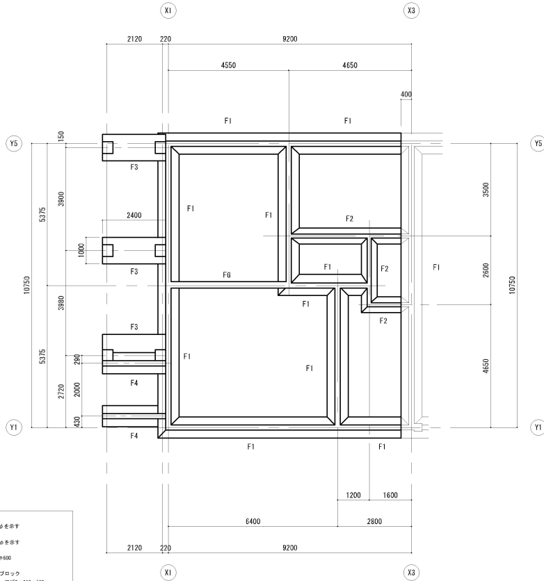
基礎架図 1/100
