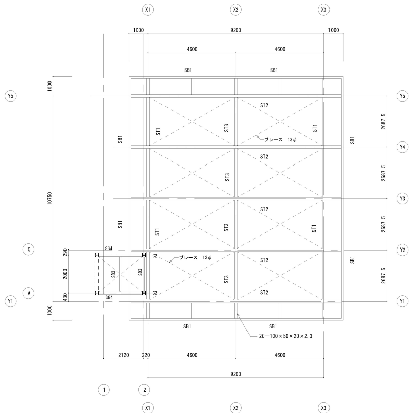
小梁架図（鉄骨部分）1/100
