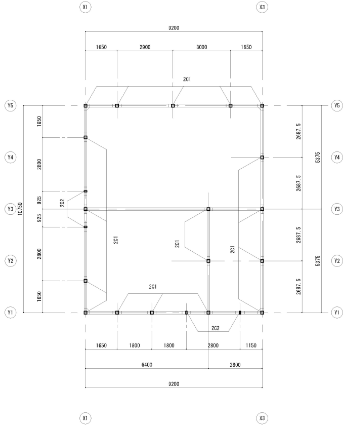
柱架図（鉄骨部分）1/100
