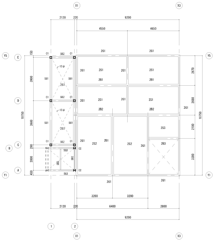
2階 梁架図 1/100
