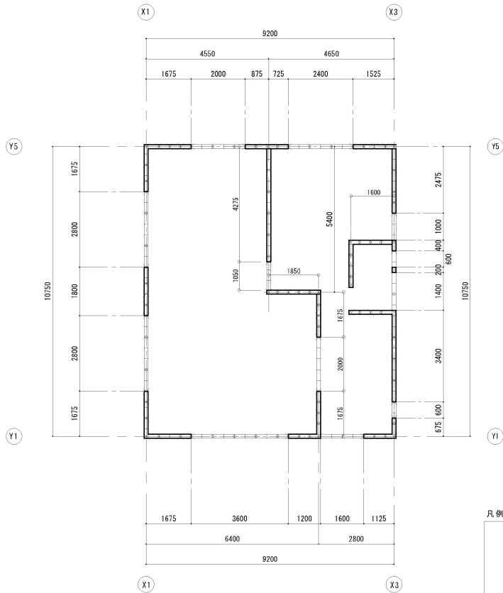
床架図（コンクリートブロック） 1/100
